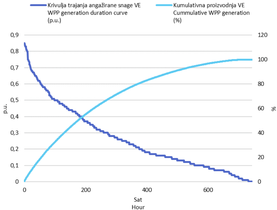
Slika 3 Krivulja trajanja angažirane snage svih VE i kumulativna proizvodnja VE u prosincu 2022. godine u jediničnim vrijednostima
