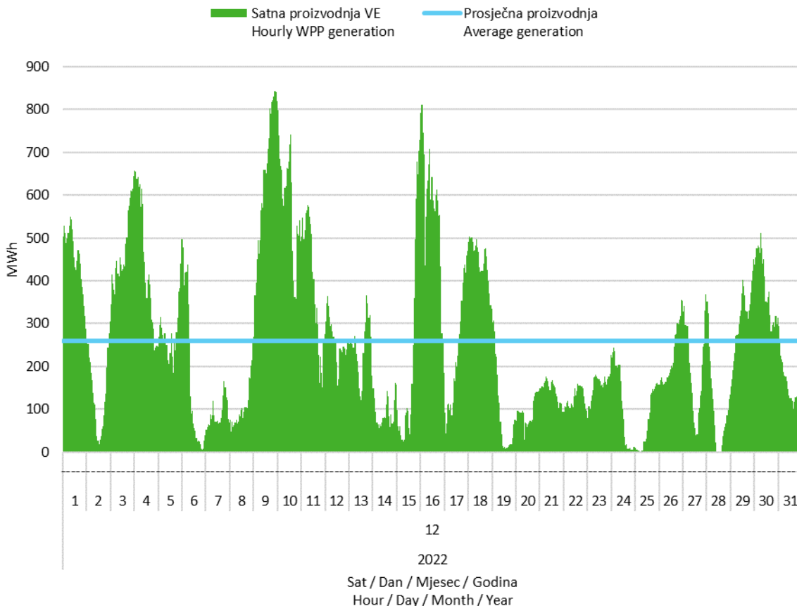
Slika 2 Satna proizvodnja svih vjetroelektrana u prosincu 2022. godine
