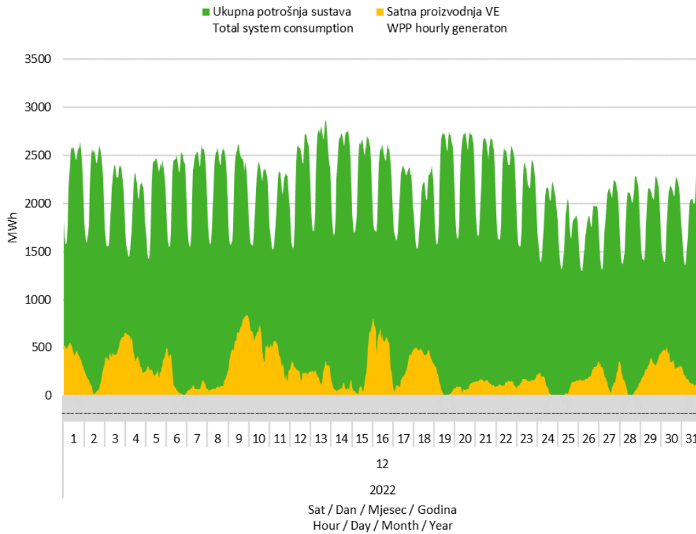
Slika 7 Usporedba satnog dijagrama opterećenja sustava i proizvodnje vjetroelektrana u prosincu 2022. godine
