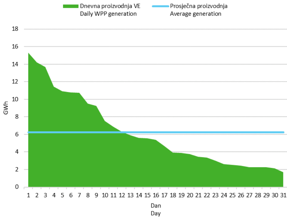
Slika 6 Krivulja trajanja dnevne proizvodnje vjetroelektrana u prosincu 2022. godine
