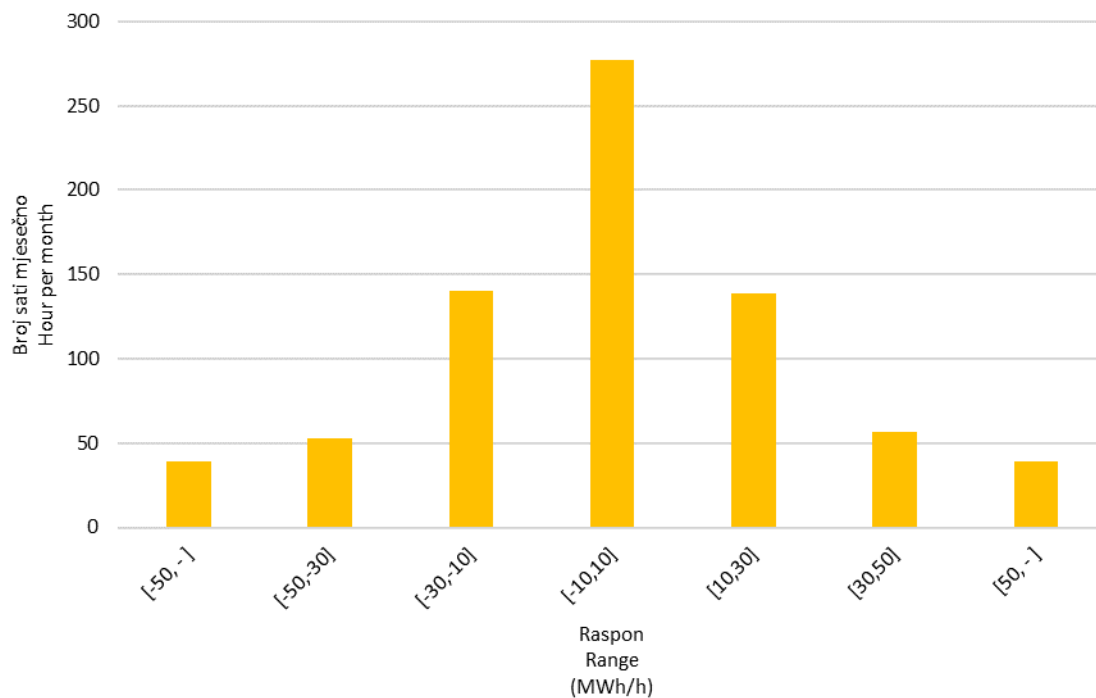
Slika 10 Statistička raspodjela satnih promjena proizvodnje VE u prosincu 2022. godine Figure 10 Statistical distribution of WPP hourly output variations in December 2022
