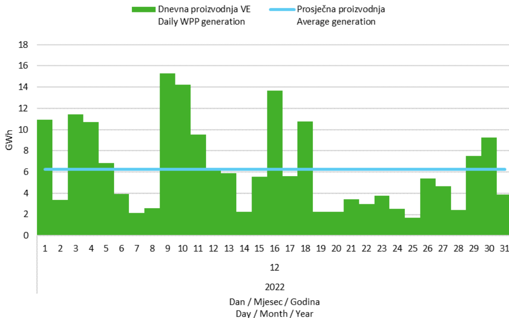
Slika 5 Dnevna proizvodnja svih vjetroelektrana u prosincu 2022. godine
