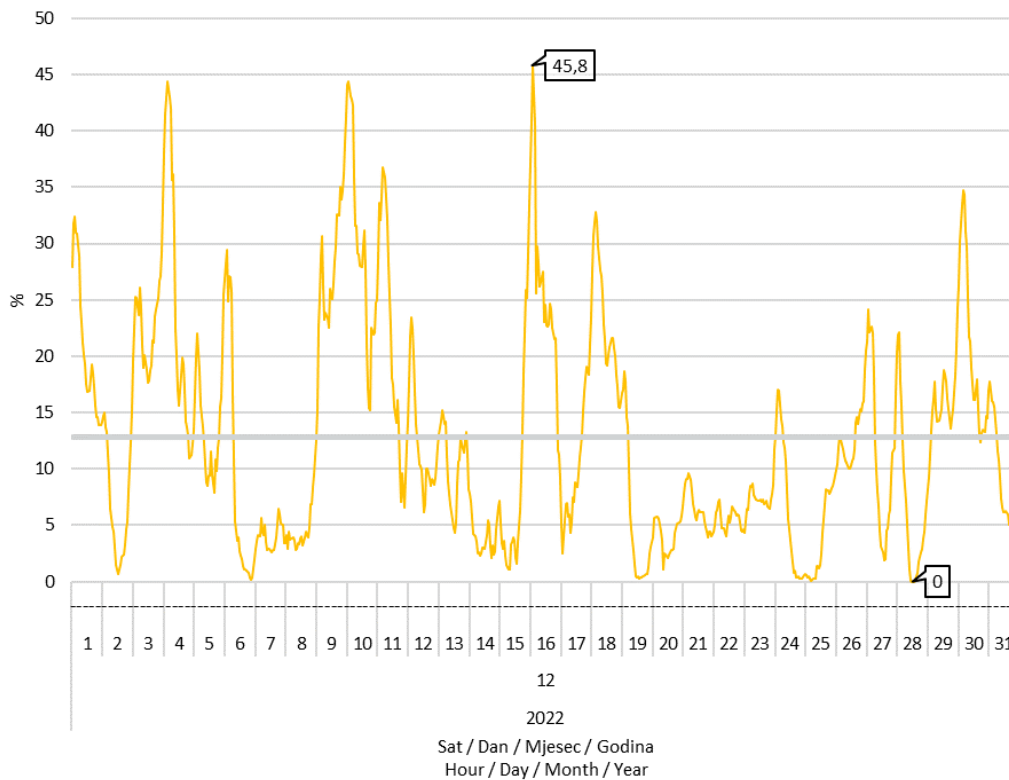
Slika 8 Udio proizvodnje vjetroelektrana u pokrivanju satnog opterećenja elektroenergetskog sustava u prosincu 2022. godine
