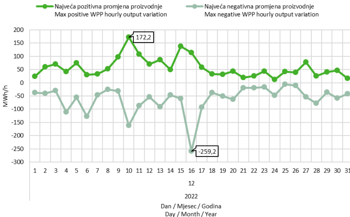
Slika 9 Maksimalna pozitivna i maksimalna negativna promjena satne proizvodnje VE u prosincu 2022. godine
